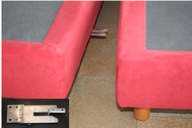
Metall-Verbindungsbeschlag
